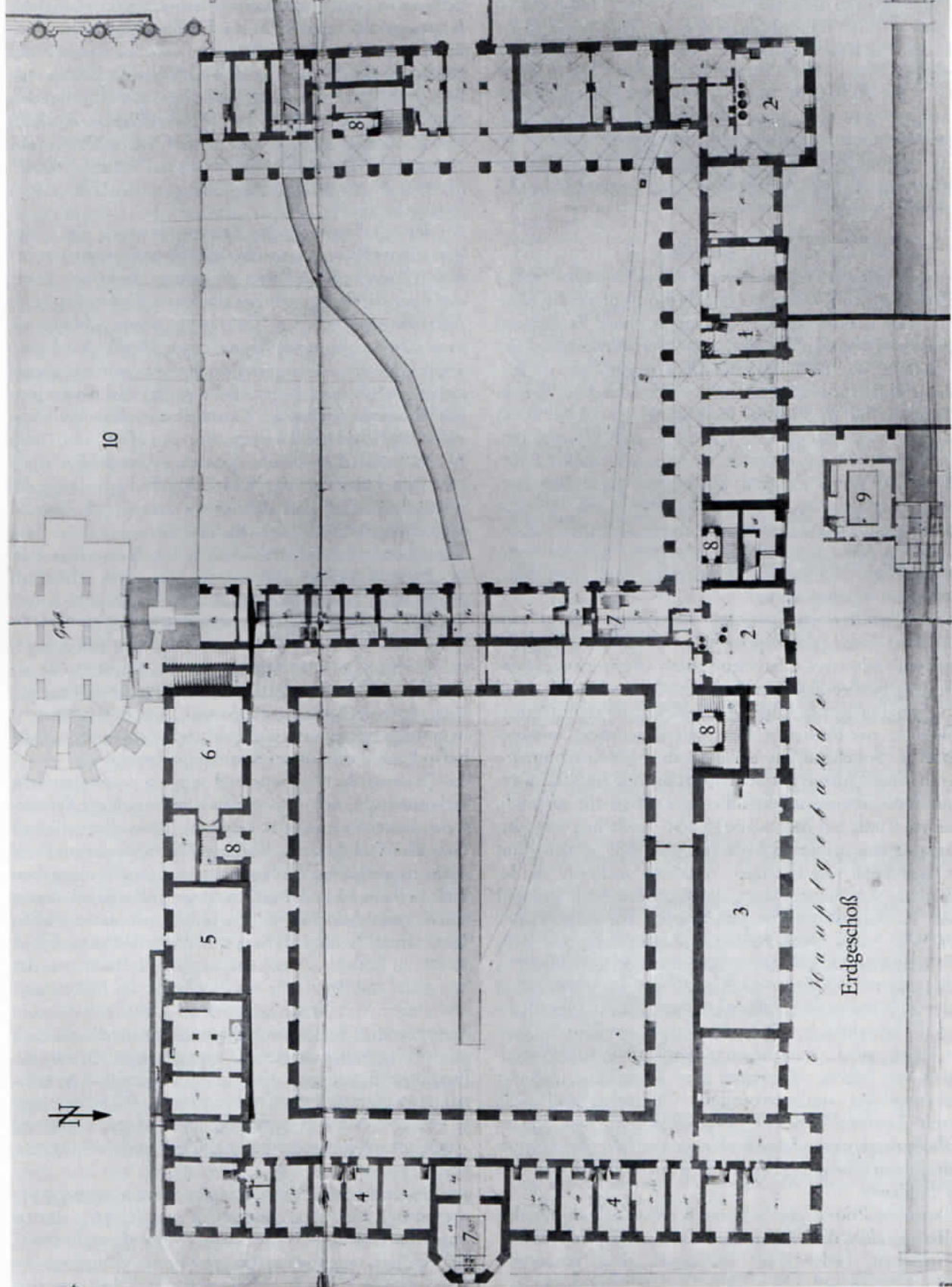
Abb. 5: Grundriß vom Erdgeschoß des Klosters Fürstfeld, Ausschnitt aus einem Plan von 1817 (Bayerisches Hauptstaatsarchiv München, Abt. IV.: Kriegsarchiv, Plansammlung Fürstfeldbruck Nr. 1), mit zusätzlichen Eintragungen: 1 Pforte – 2 Küchen – 3 Refektorium – 4 Zellen der Laienbrüder – 5 Noviziat – 6 Kapitelsaal – 7 Abortanlagen – 8 Treppenhäuser – 9 Fischkalter – 10 Klosterkirche.
