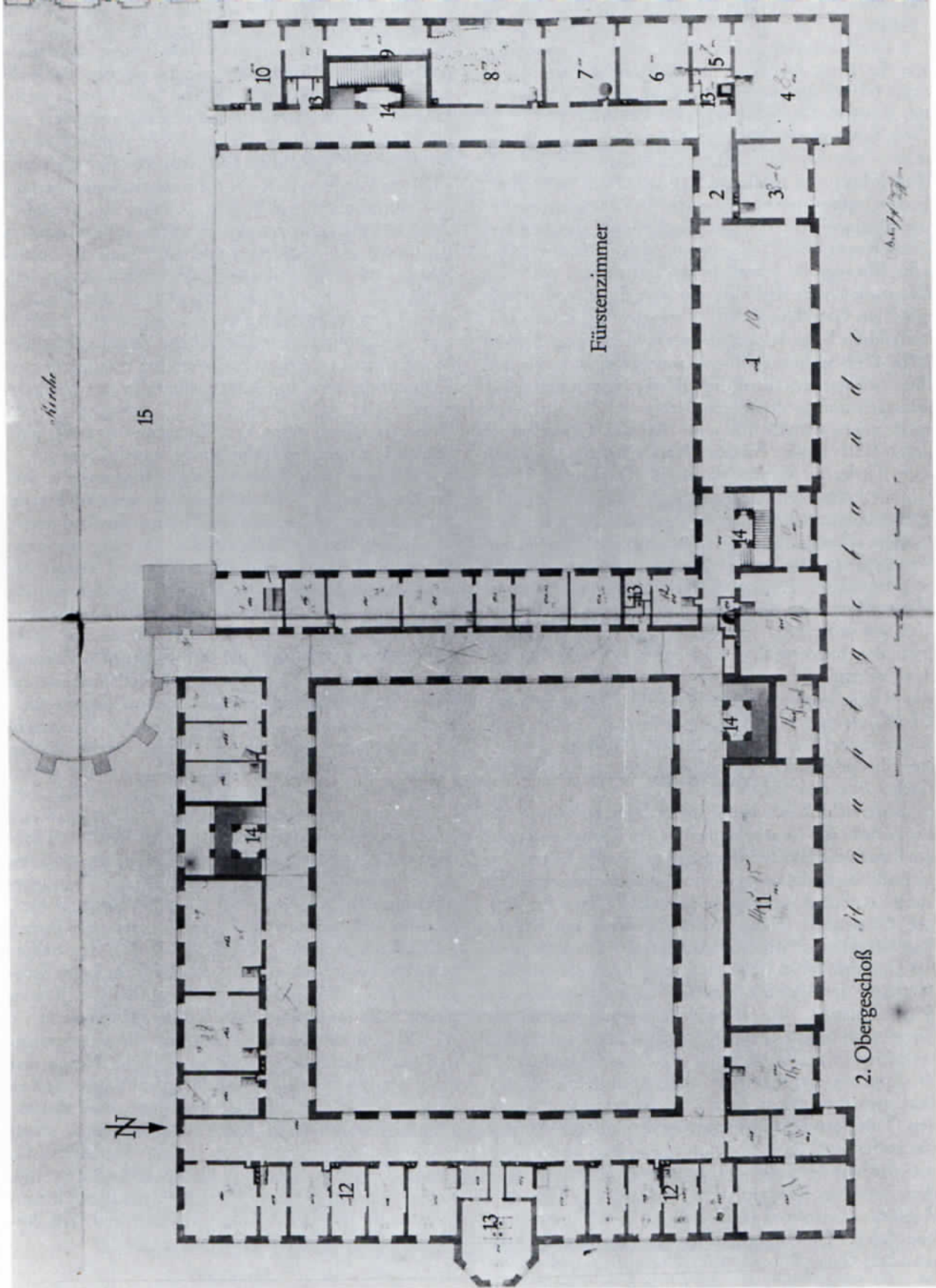
Abb. 3: Grundriß vom 2. Obergeschoß des Klosters Fürstenfeld, Ausschnitt aus einem Plan von 1817 (Bayerisches Hauptstaatsarchiv München, Abt. IV: Kriegsarchiv, Plansammlung Fürstenfeldbruck Nr. 3), mit zusätzlichen Eintragungen: 1 Fürstensaal – 2 Vorflöz – 3 »Persenes« Zimmer – 4 Kurfürstliches Speisezimmer – 5 Kurfürstliche Kapelle – 6 Zimmer der Kurfürstin – 7 Zimmer des Kurfürsten – 8 Gelbes Zimmer – 9 Billardzimmer – 10 Blaues Zimmer – 11 Klosterbibliothek – 12 Gästezimmer des Klosters – 13 Abortanlagen – 14 Treppenhäuser – 15 Klosterkirche.
