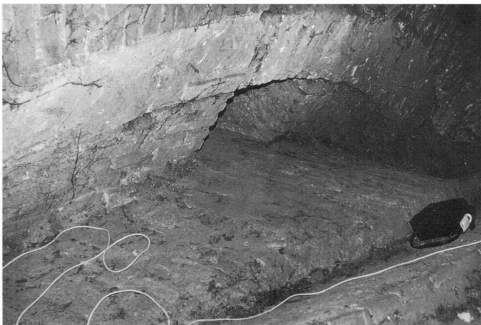
St. Peter und Paul in Neustift: Mauerwerk des Gurtbogens einer Seitenkapelle vor 1751. Darunter Einstieg in den Gewölbehohlraum.
