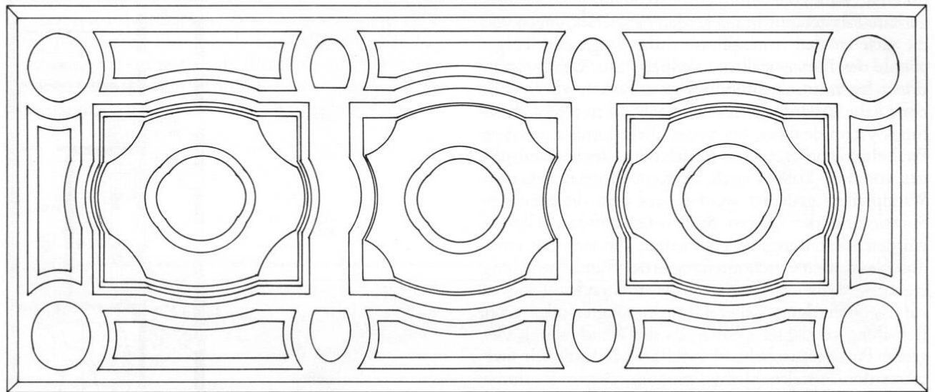
Abb. 7a und 7b: Aufmaßzeichnung eines Deckenspiegels, gezeichnet 1909 von Hermann Mader, darunter die schematische Anpassung an die Maße des Fürstensaales durch Verzerrung der Breite. Foto u. Zeichnung: Langosch, Büro Zeh, Jesenwang
